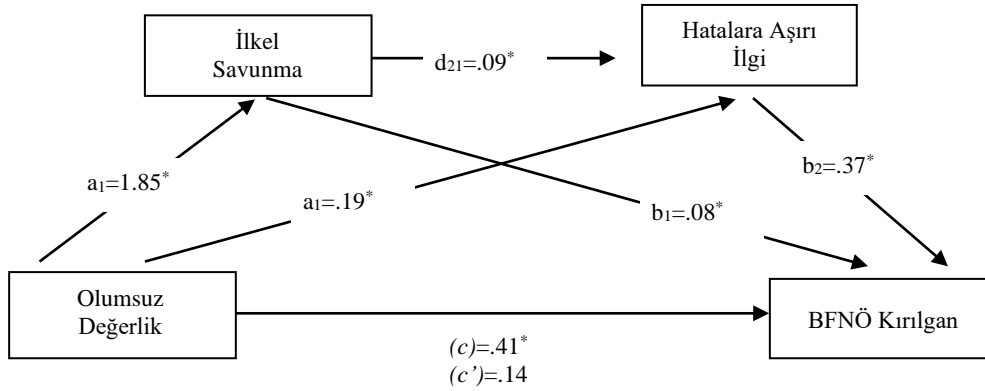
Şekil 3. Olumsuz Değerlik ve Kırılgan Narsisizm Arasındaki İlişkide İlkel Savunma Grubu ve Hatalara Aşırı İlgi Değişkenlerinin Seri Çoklu Aracılık Etkisi
